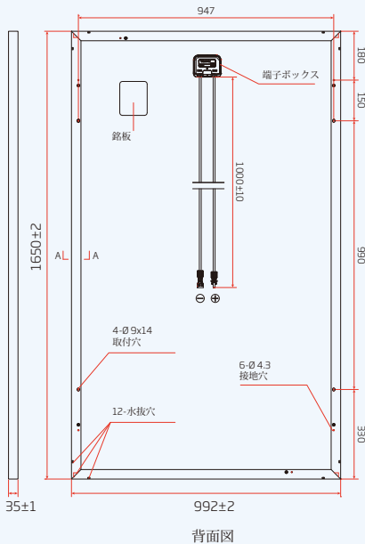
背面図
